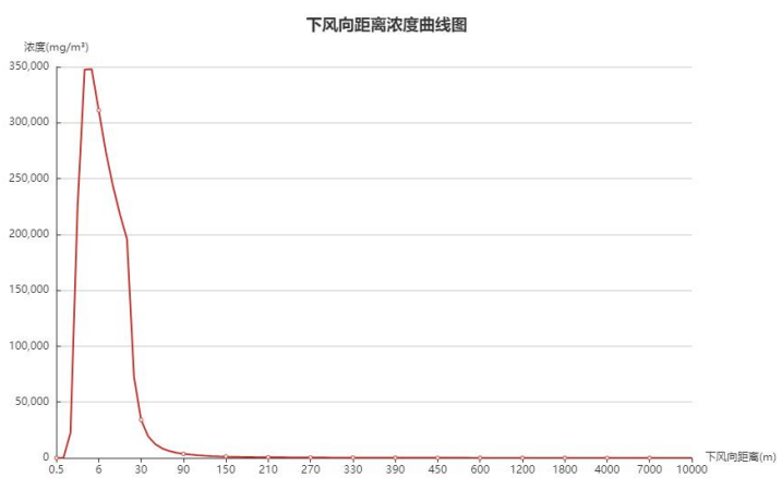
图 6.5-24 LNG 泄漏燃烧次生 CO 扩散最不利气象最大浓度-距离曲线图
