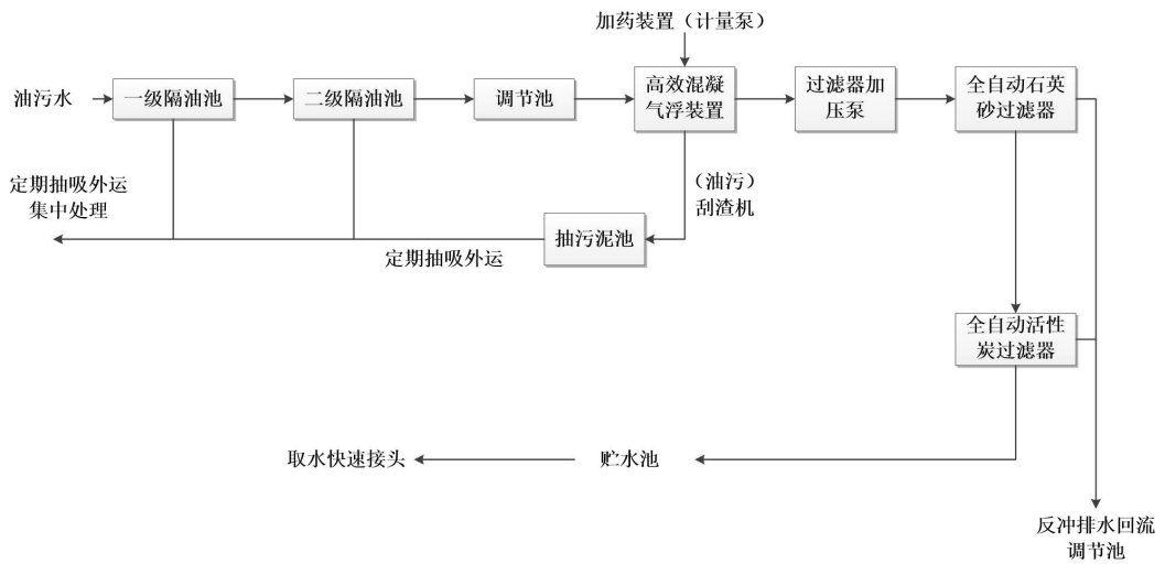
图 5.3-2 小漠港一期工程油污水处理系统工艺流程图
