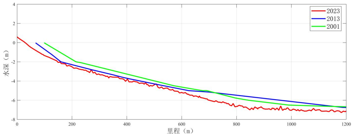
图 4.1-13 断面 3 剖面地形对比
