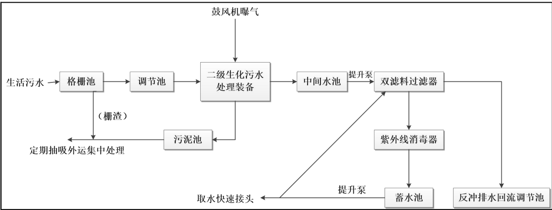
图 3.1-10 生活污水处理工艺流程图
