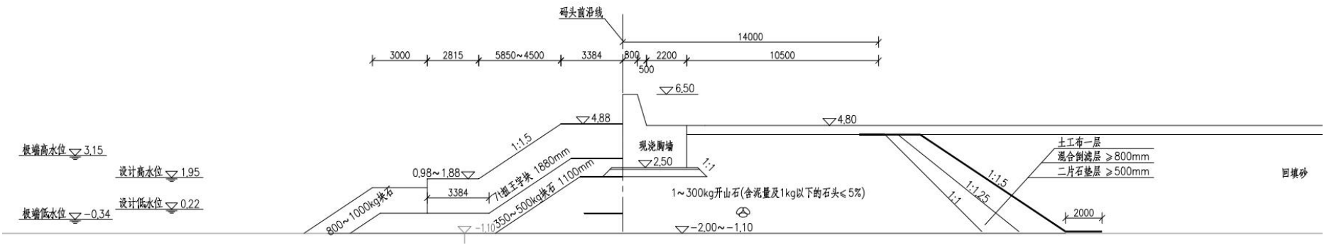
图 3.1-6 浅滩段东侧护岸典型断面图
