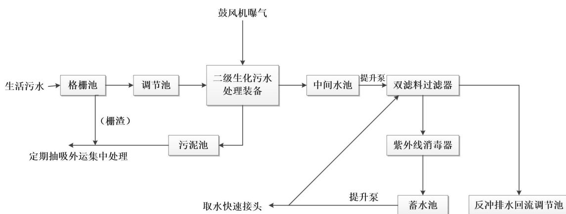
图 7.4-1 小漠港一期工程生活污水处理站工艺流程图
