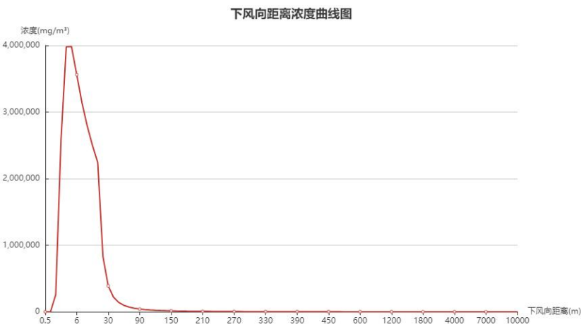
图 6.5-22 LNG 泄漏甲烷扩散最不利气象最大浓度-距离曲线图
