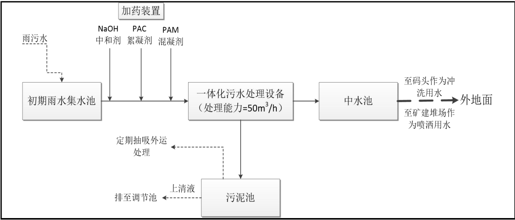
图 5.3-1 小漠港一期工程初期雨水处理系统工艺流程图
