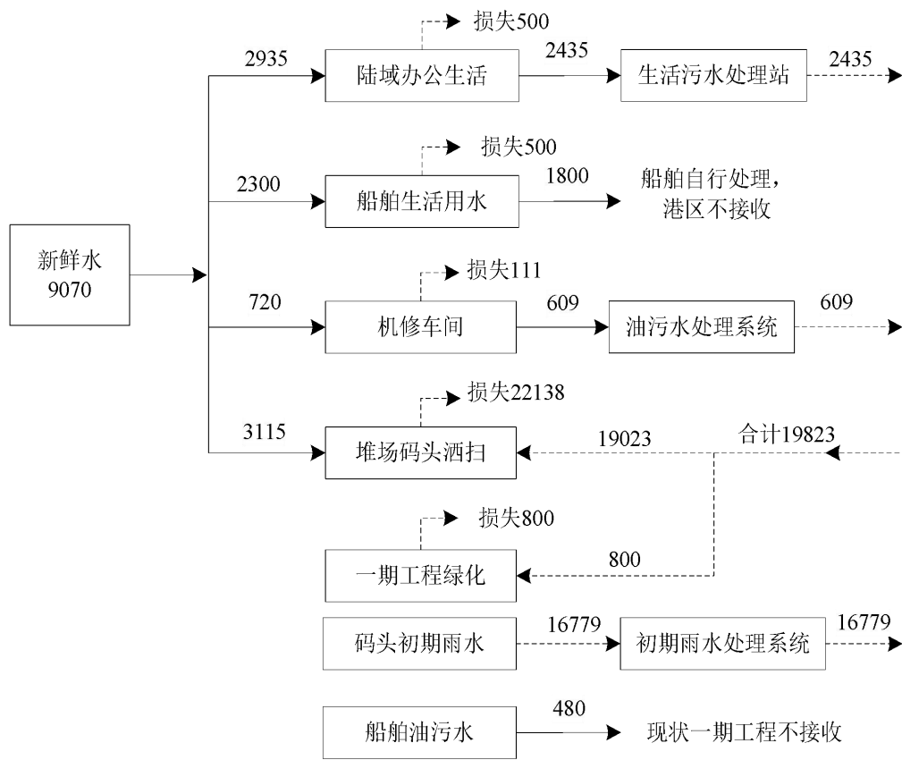
图 3.1-7 现有项目水平衡图
