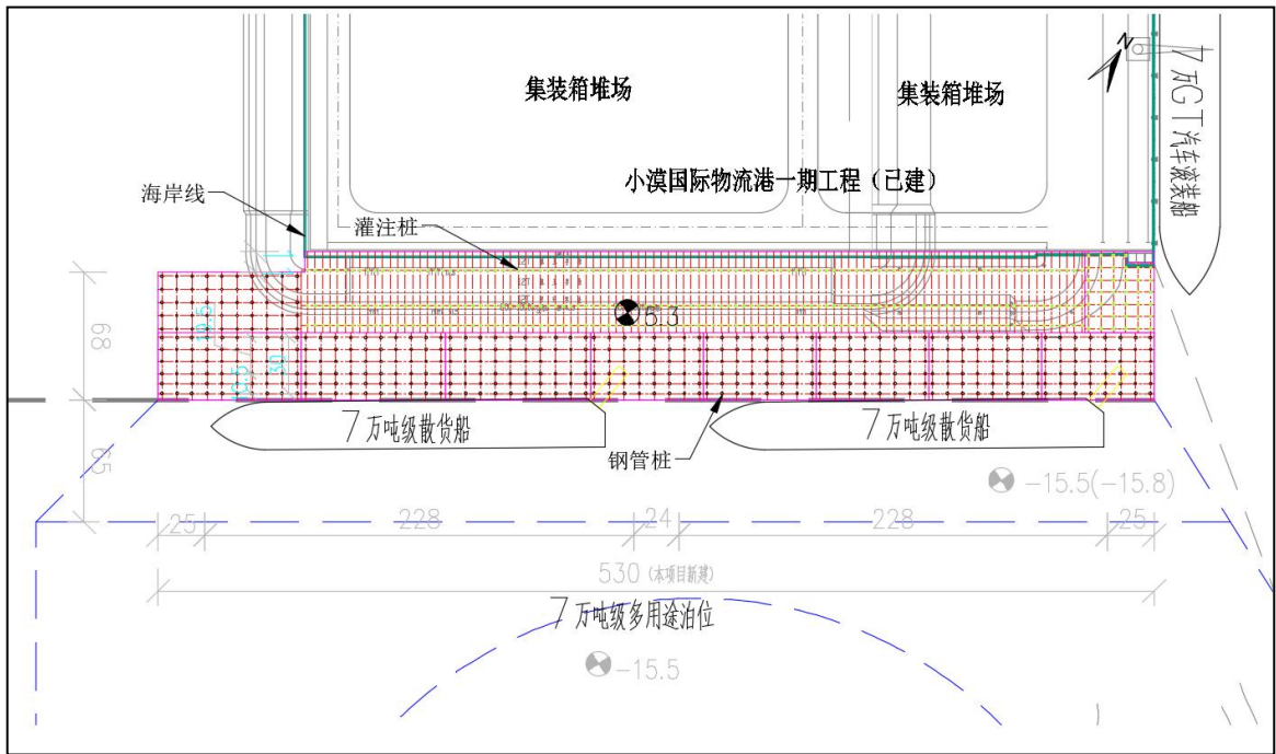
图 3.2-7b 码头平面方案桩基位置图
