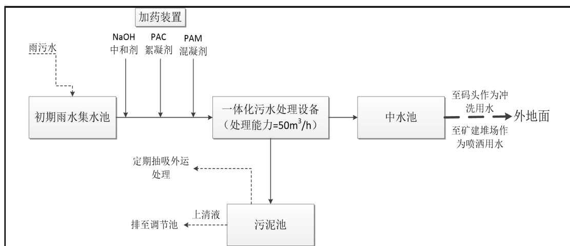
图 3.1-8 系统 1 初期雨水处理工艺流程图
