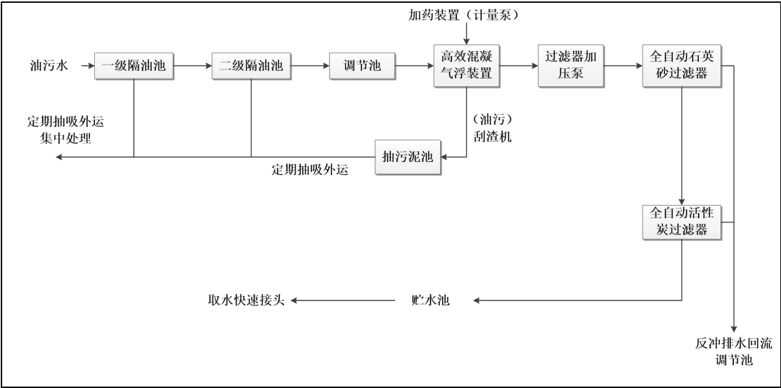
图 3.1-9 系统 2 含油污水处理工艺流程图
