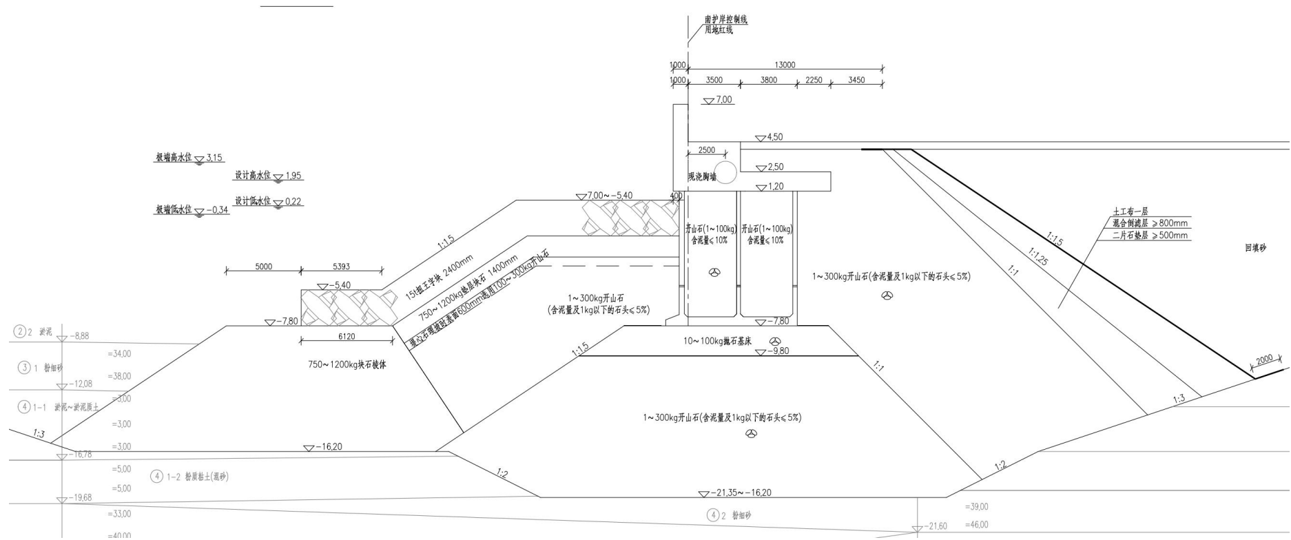
图 3.1-4 南段护岸及部分西侧护岸典型断面图
