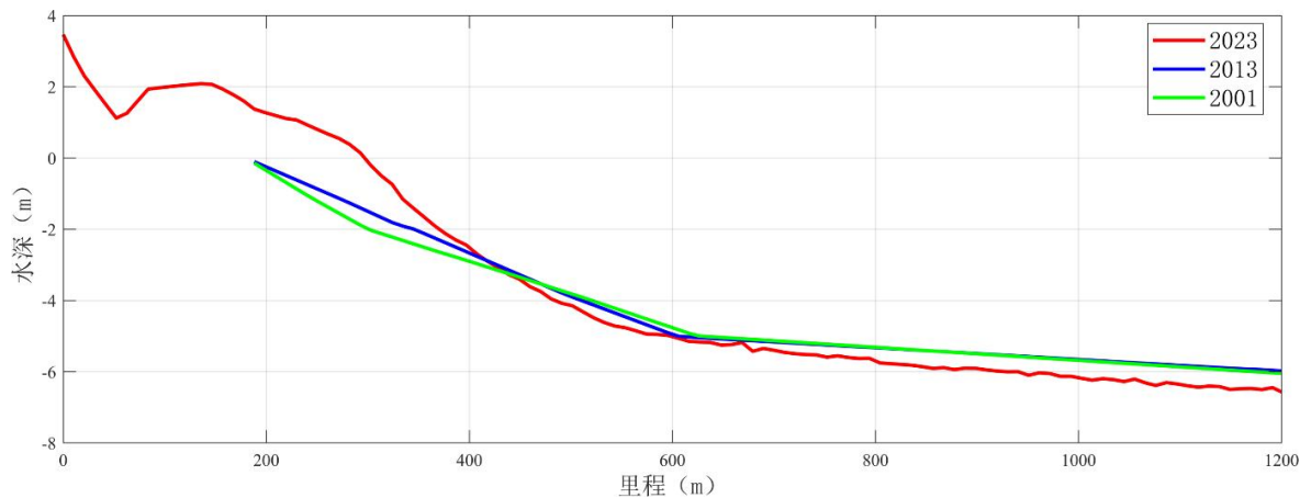
图 4.1-11 断面 1 剖面地形对比
