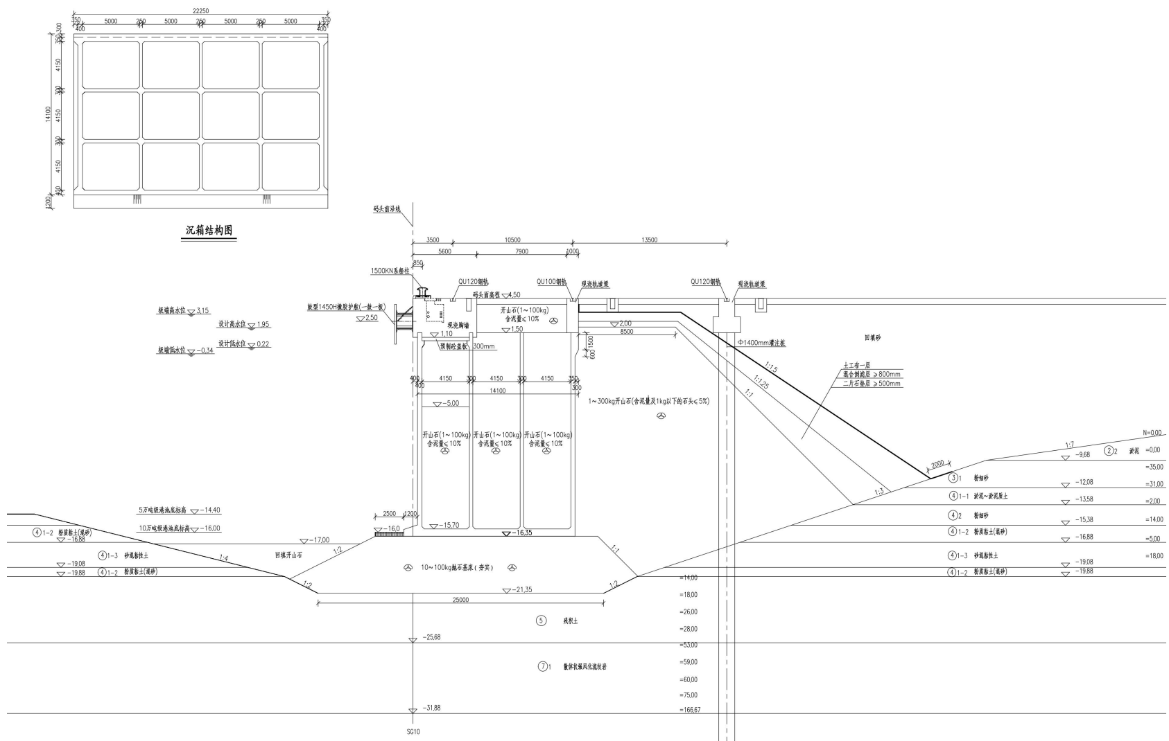
图 3.1-2 多用途码头泊位码头结构断面图
