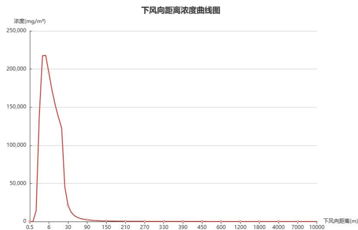
图 6.5-28 LNG 泄漏燃烧次生 CO 扩散最常见气象最大浓度-距离曲线图
