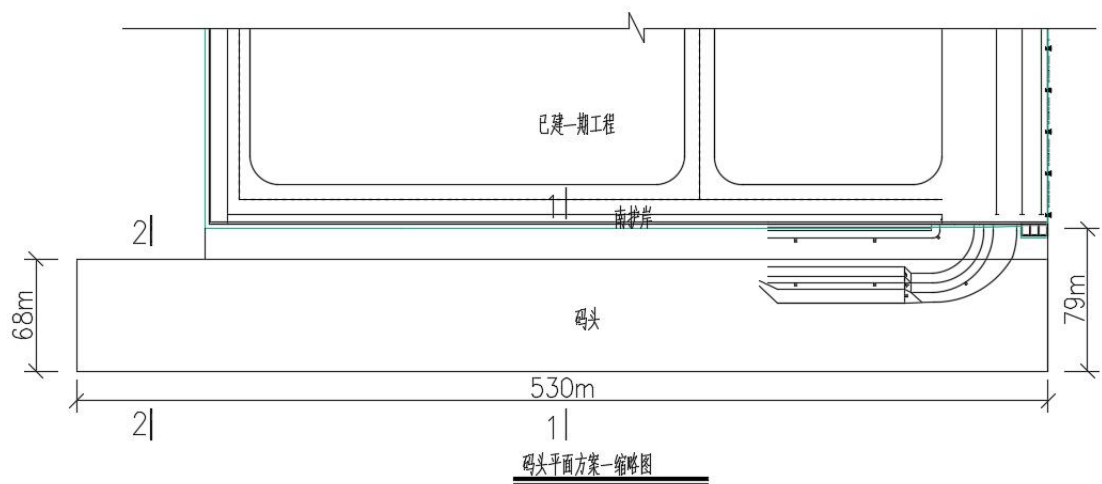
图 3.2-7a 码头平面方案缩略图
