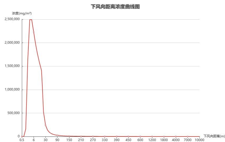
图 6.5-26 LNG 泄漏甲烷扩散最常见气象最大浓度-距离曲线图
